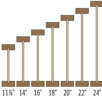
PWI 90 7/16" OSB Web 3 1/2" x 1 1/2" Flange
